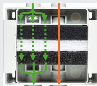
TX-LFx-2-W Filterwirkung Kanal 2
