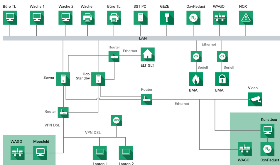
Topologieübersicht VisuLAN System im Lenbachhaus
